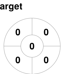
BRIS2
