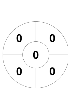
BRIS2
